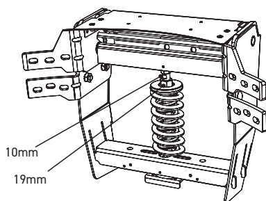
BISAGRA ALTERNATIVA
