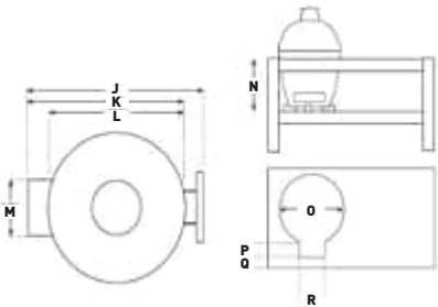
VISTA DALL'ALTO
