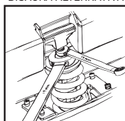
BISAGRA ALTERNATIVA
