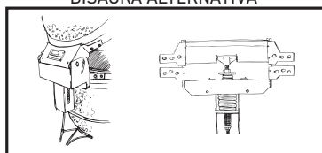
BISAGRA ALTERNATIVA
